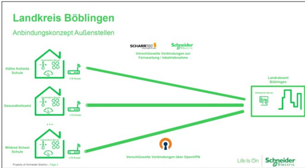
Abbildung 5: Anbindungskonzept Außenstellen
